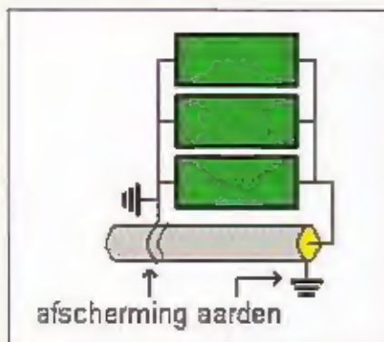
Figuur 5. De afscherming van de coaxkabel wordt dicht mogelijk bij het aardpunt van de dummyload-weerstanden gead, maar de coaxkabel loopt nog verder door tot aan de 'bete' aansluiting.
